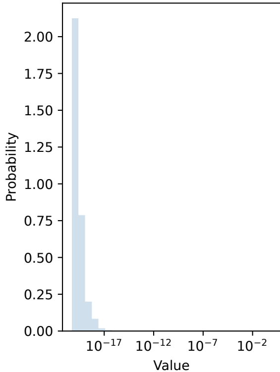
1e17 Posterior
