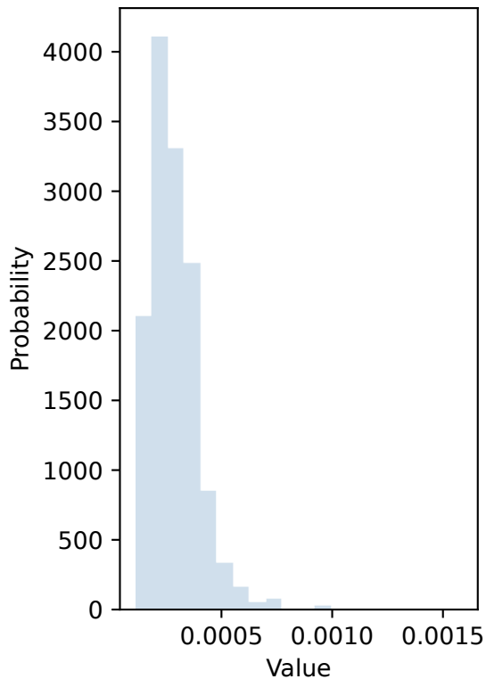
Posterior
