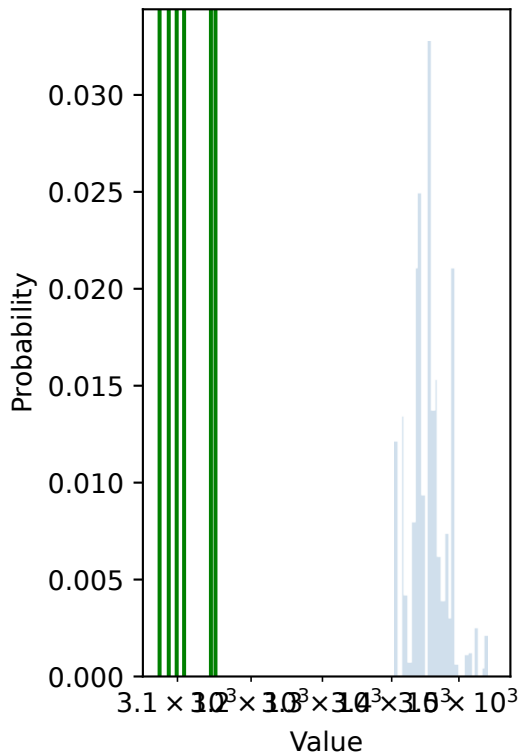
Posterior
