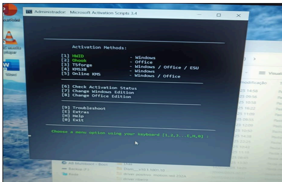
Figura 9 - Software
