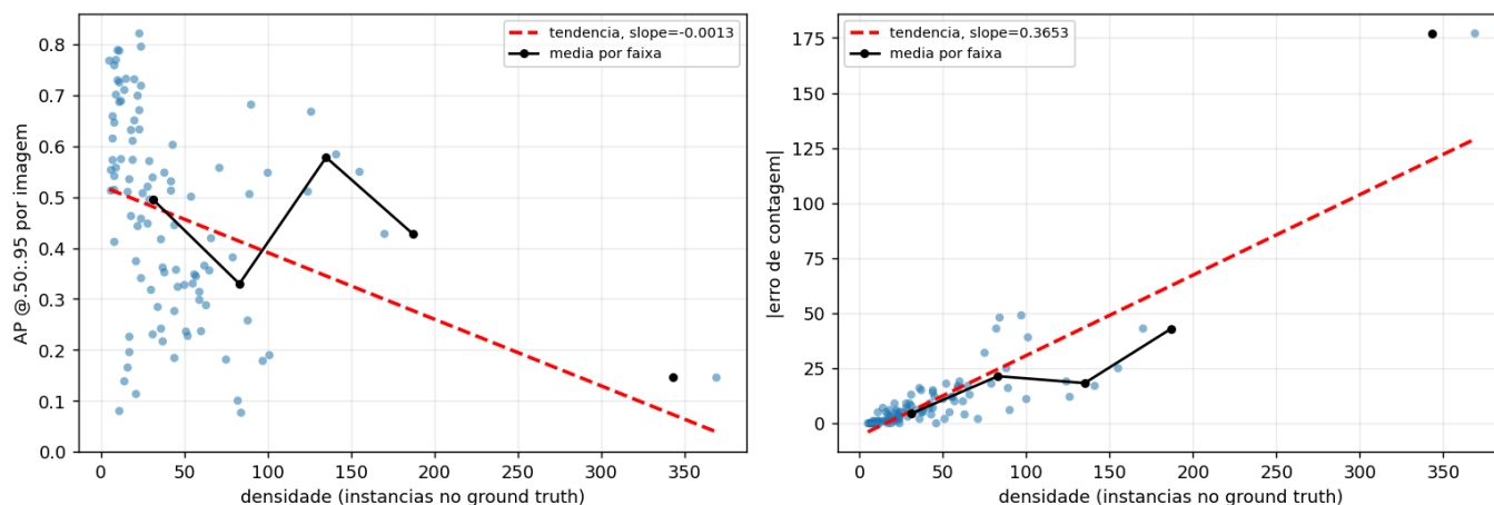
dsb2018_baseline: mAP e erro de contagem contra densidade
