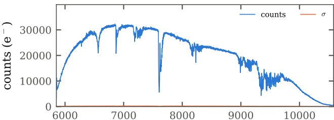
slit 705, median S/N per pixel 123.9
