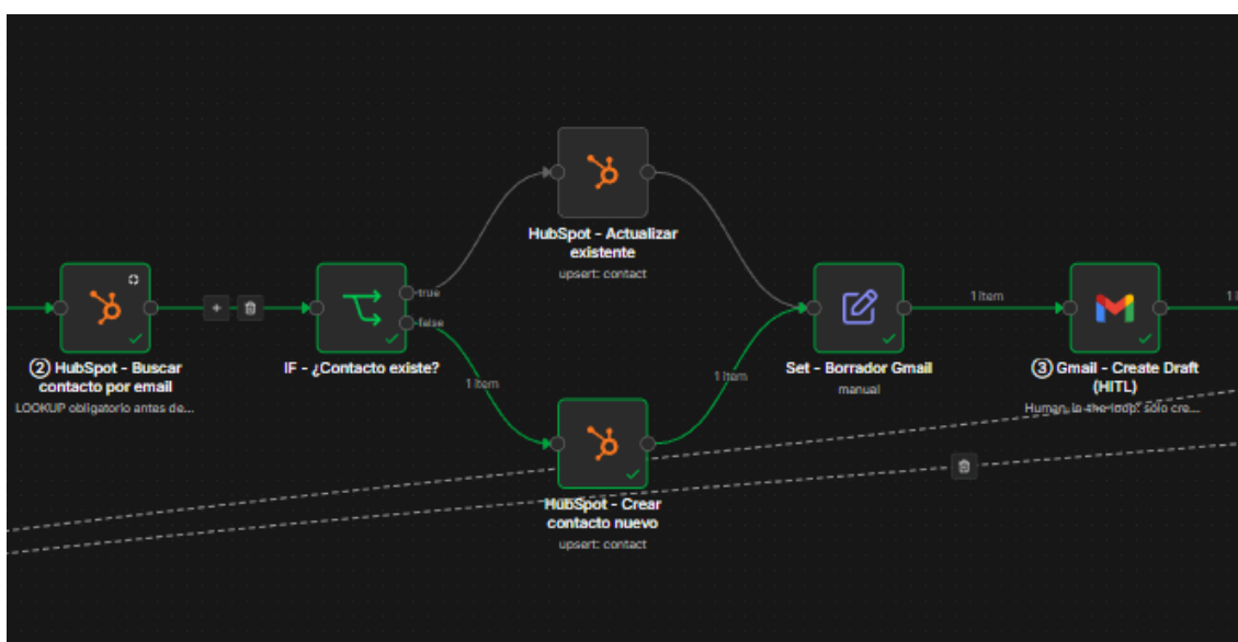
Figura 4. Contacto nuevo: Lookup → FALSE → Crear contacto nuevo.
