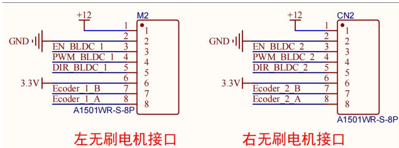
图 3-7 电机驱动电路
