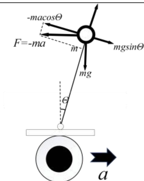
图 1-3 施加加速度后物理模型
