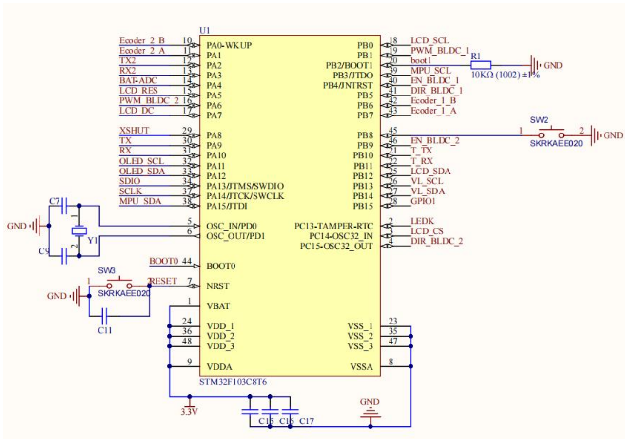
图 3-2 STM32 最小系统
