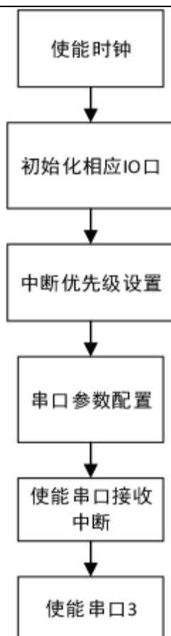
图 4-6 串口 3 初始化
