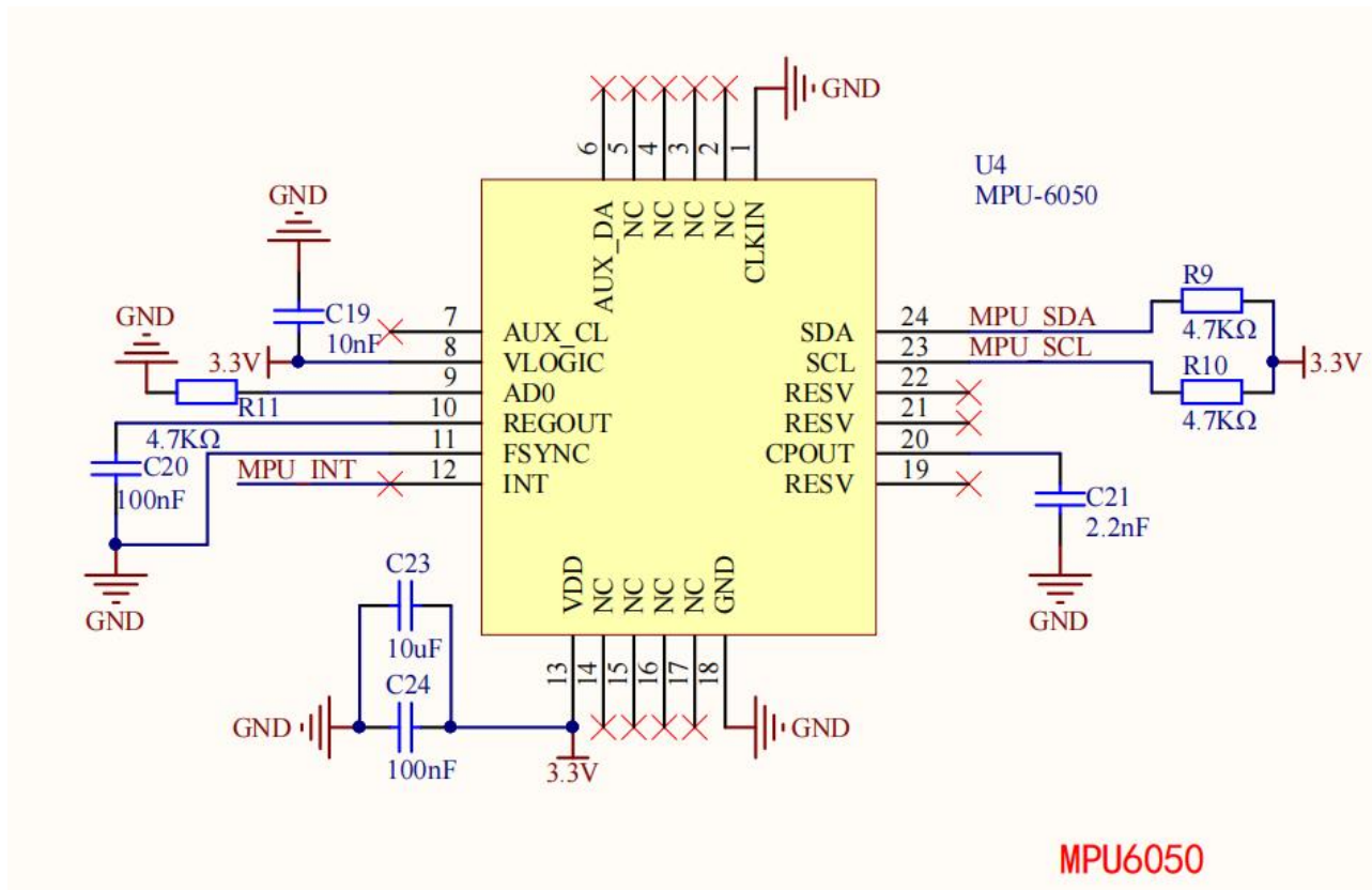
图 3-6 MPU6050 模块原理图
