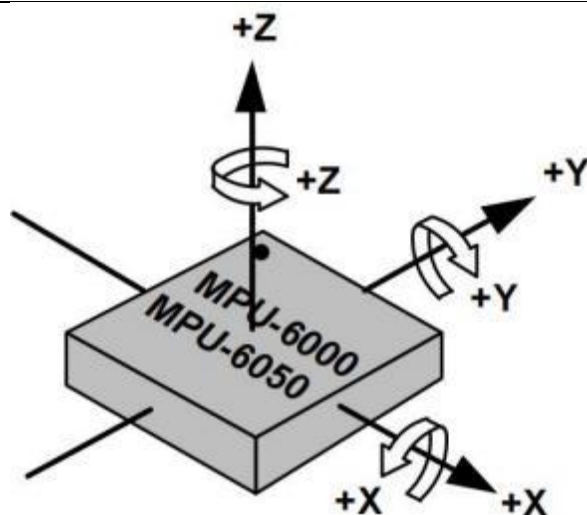
图 2- 1 MPU6050 坐标系
