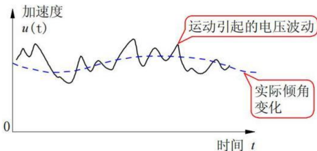
图 2-3 测量倾角与实际倾角对比
