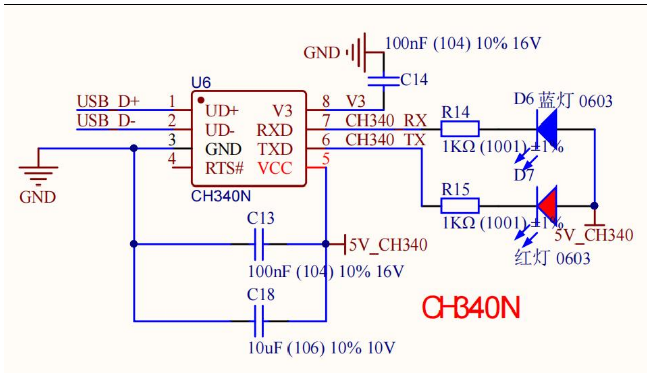
图 3-3 USB 转 TTL 电路
