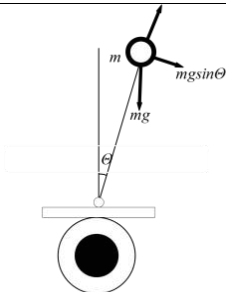
图 1-2 小车倾斜受力分析
