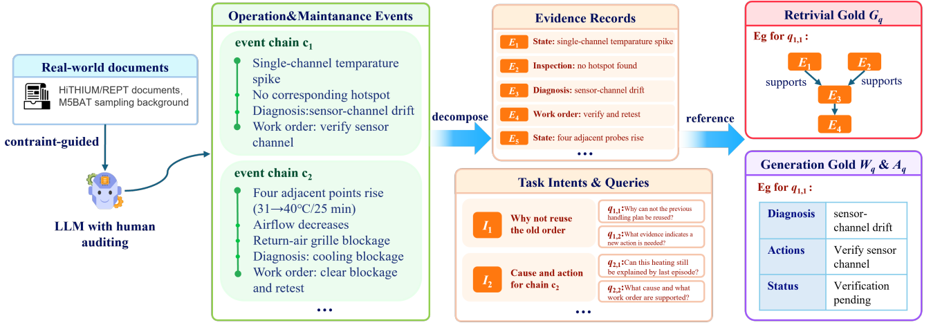
Fig. 2. TEF-RAG v6 Semantic Benchmark v1 的构建流程与示例。公开资料用于约束设备与数据背景；在此基础上构造运维事件链 c ，并派生证据记录 e_i 、任务意图 I_j 与查询 q_{j,p} 。随后针对具体查询分别建立检索参考证据流与结构化生成参考答案，用于检索和下游生成评价。
