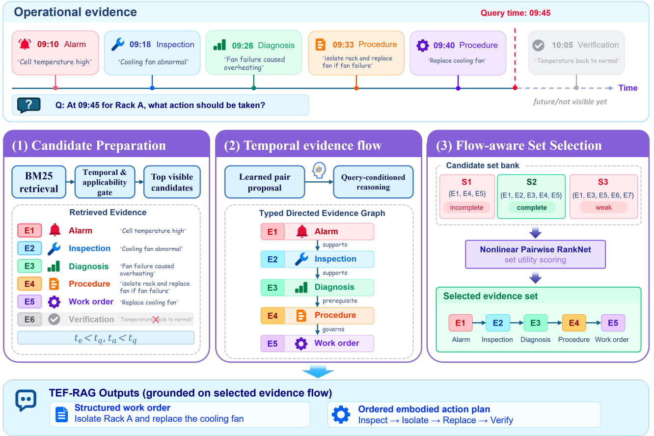
Fig. 1. TEF-RAG 总体框架。系统先从查询时刻合法的候选证据中构建查询条件化的时序证据图，再对候选证据集合进行非线性 pairwise ranking，以恢复完整的 Top-5 evidence flow；该证据流随后作为受控上下文生成标准化工单与有序具身指令序列。本文 v6 封存 benchmark 重点评价图中 evidence-flow retrieval 部分。
