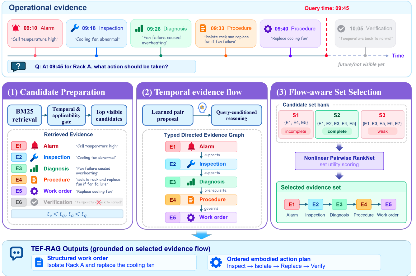
Fig. 1. TEF-RAG 总体框架。系统首先从查询时刻合法的记录中选择候选证据对，随后构建查询条件化的时序证据流。非线性成对排序器从候选集合空间中选择至多五条记录构成证据流，并将其作为受控上下文输入共享的下游生成器。
