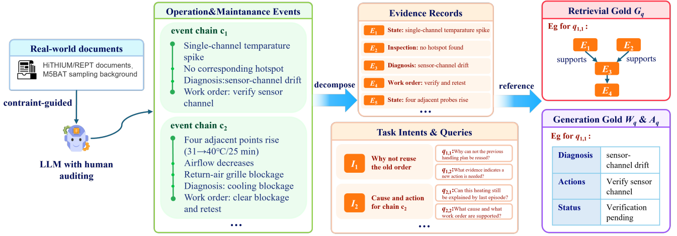
Fig. 2. TEF-RAG v6 Semantic Benchmark v1 的构建流程与示例。公开资料用于约束设备与数据背景；随后构造一条运维事件链 c ，并由其派生证据记录 e_i 、任务意图 I_j 与查询 q_{j,p} 。之后为每个查询分别构建检索参考证据流和结构化生成参考答案，用于检索与下游生成评估。
