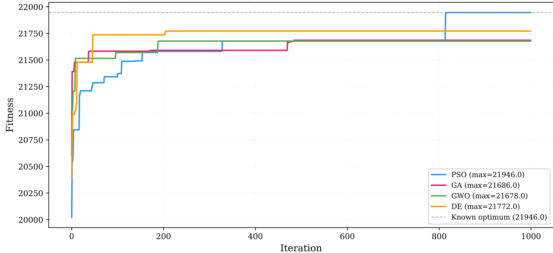
V-Explotación — All MHs (seed=1)
