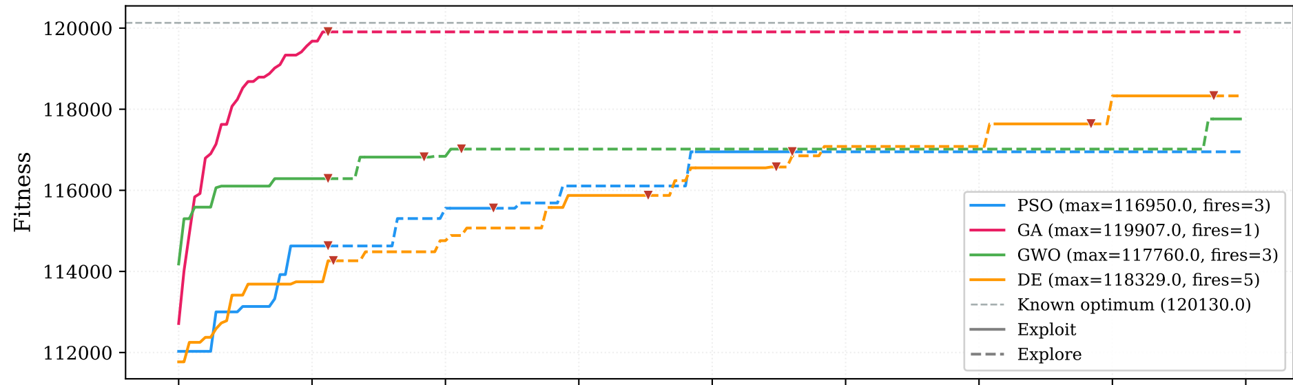
Fire D2 — All MHs (seed=1)
