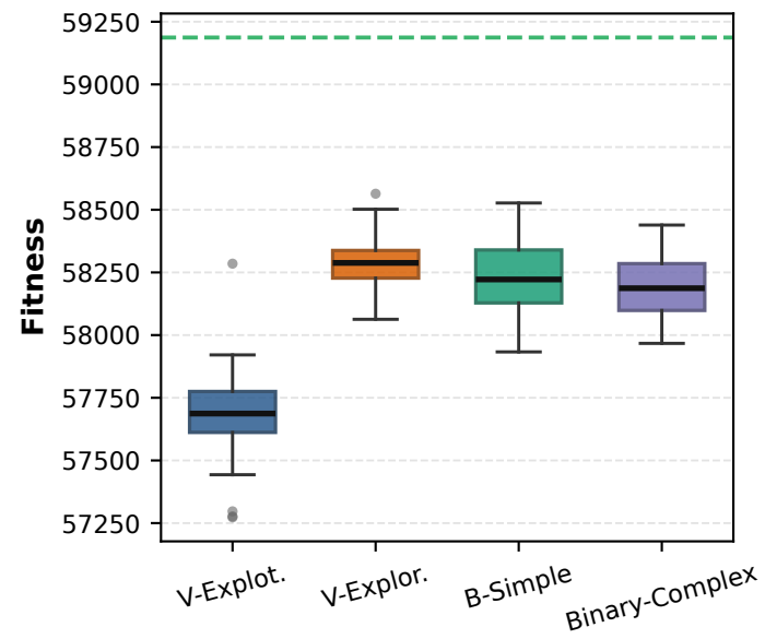
PSO
