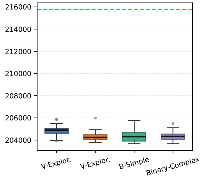
GWO
