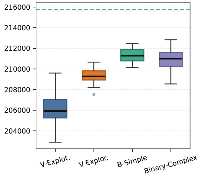
DE
