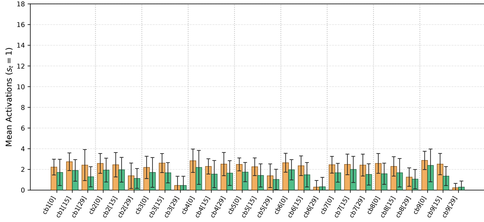
BGWO
