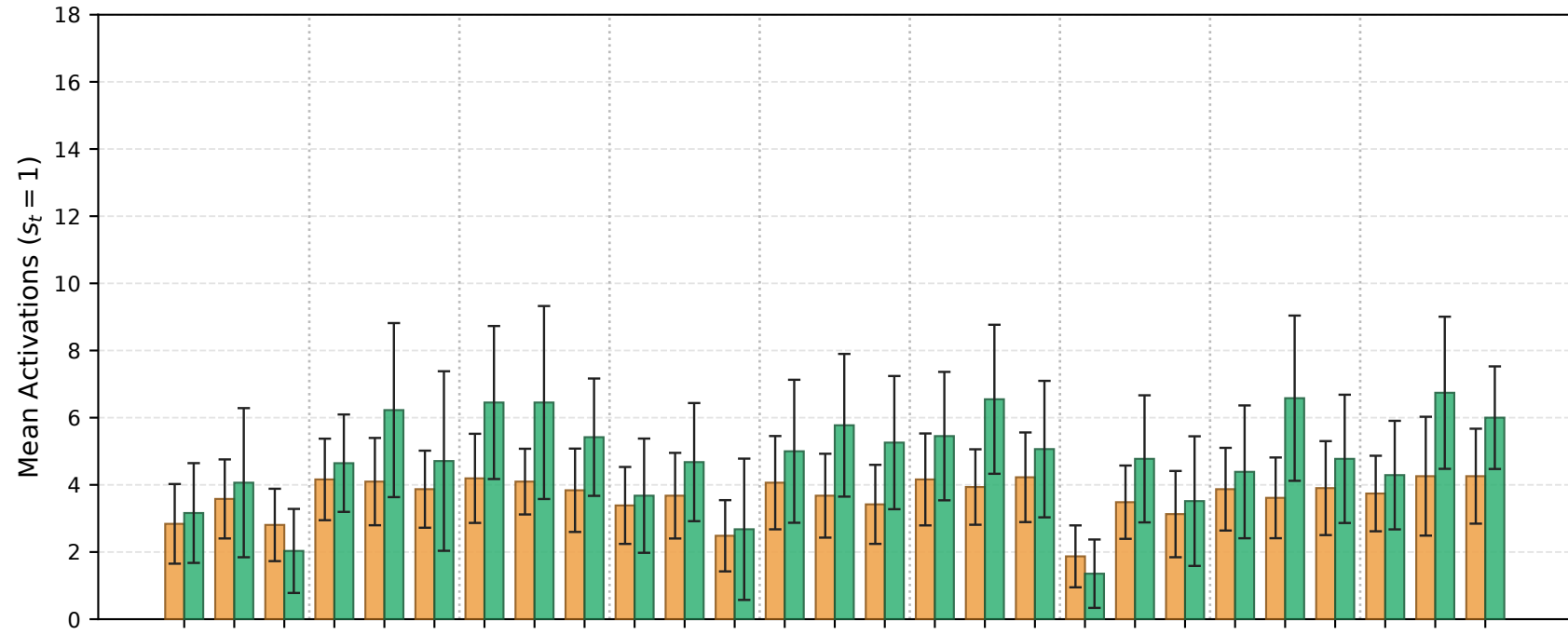
BGWO
