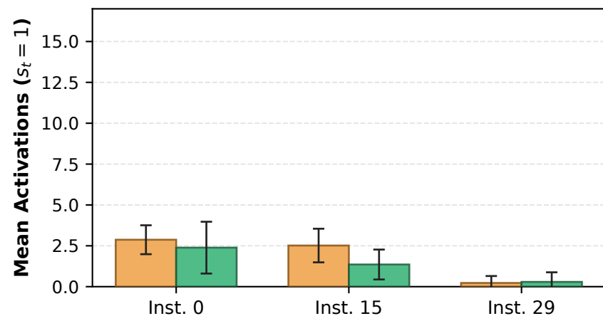
BGWO
