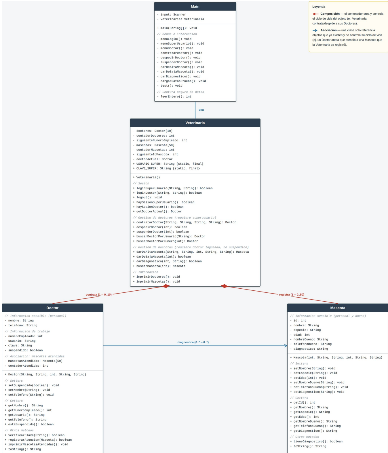
Ilustración 1: Diagrama de clases — Main, Veterinaria, Doctor y Mascota.
