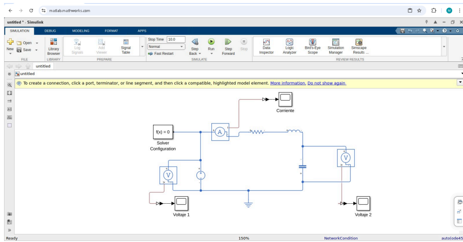
Figura 2. Circuito con bloques de simscape.
