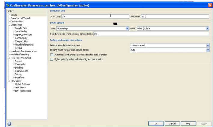
Figura 3. Ventana de parámetros de Simulink.
