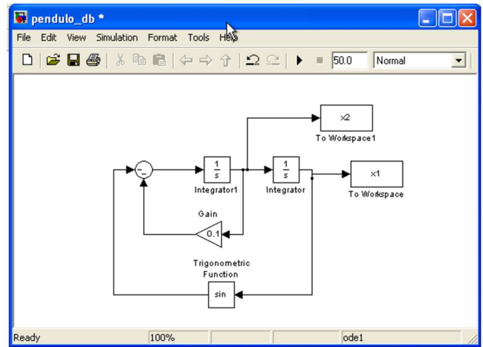
Figura 2. Diagrama de bloques en Simulink del péndulo.
