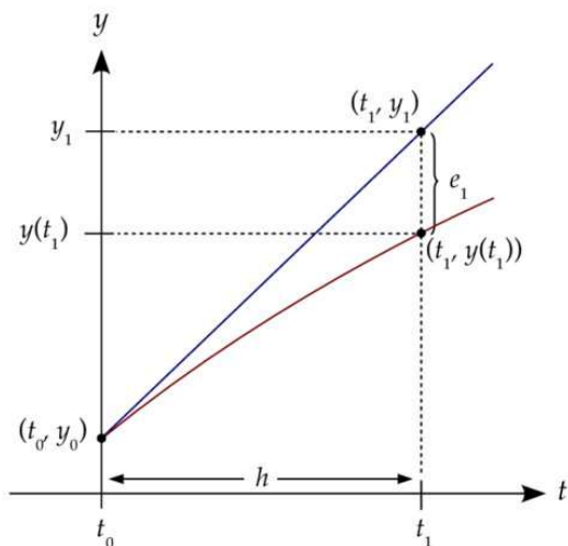
Figura 1. Interpretación geométrica del método de Euler.
