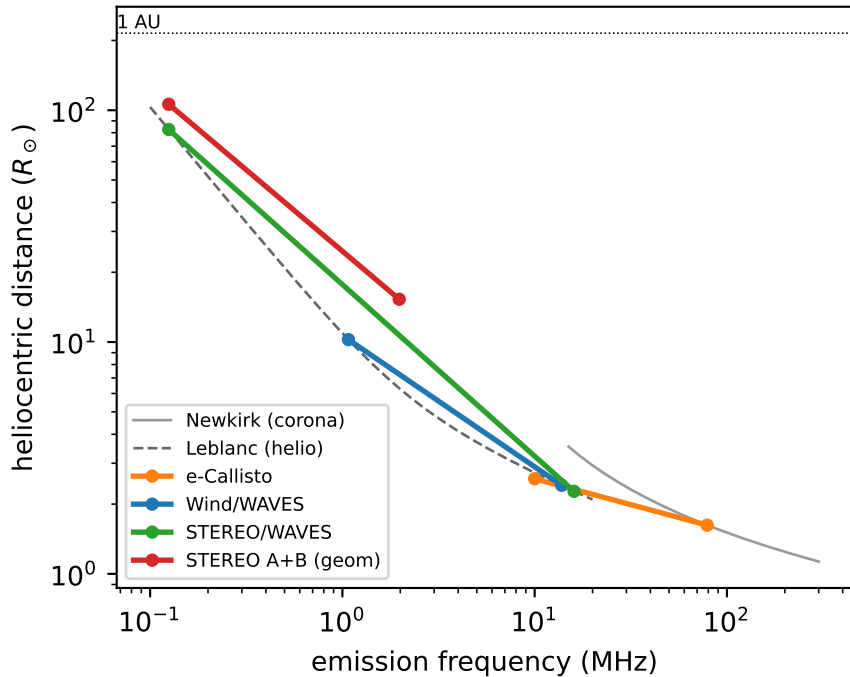
Type III beam: corona to 0.4 AU
