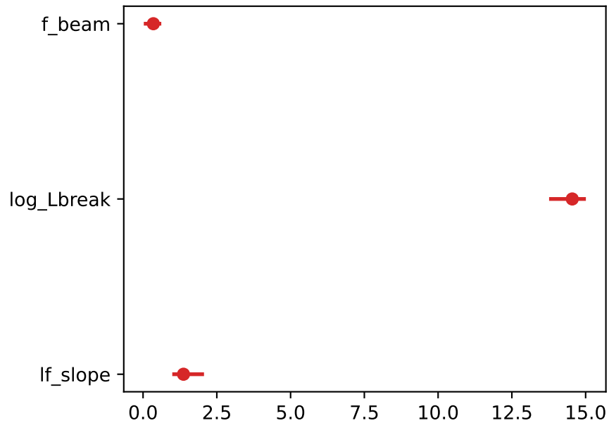
Posterior (90% CI)
