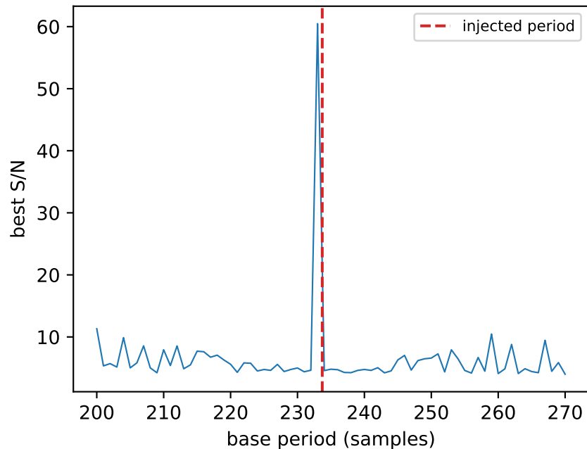
FFA periodogram
