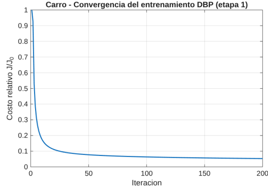
Figura 1: Convergencia del entrenamiento DBP del carro (costo relativo J/J_0 ).
