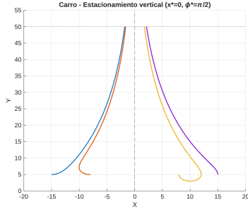
Figura 2: Estacionamiento vertical.
