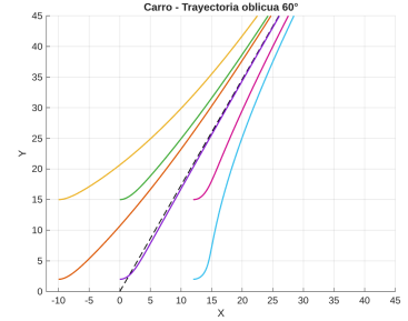
Figura 4: Oblicua 60^\circ .
