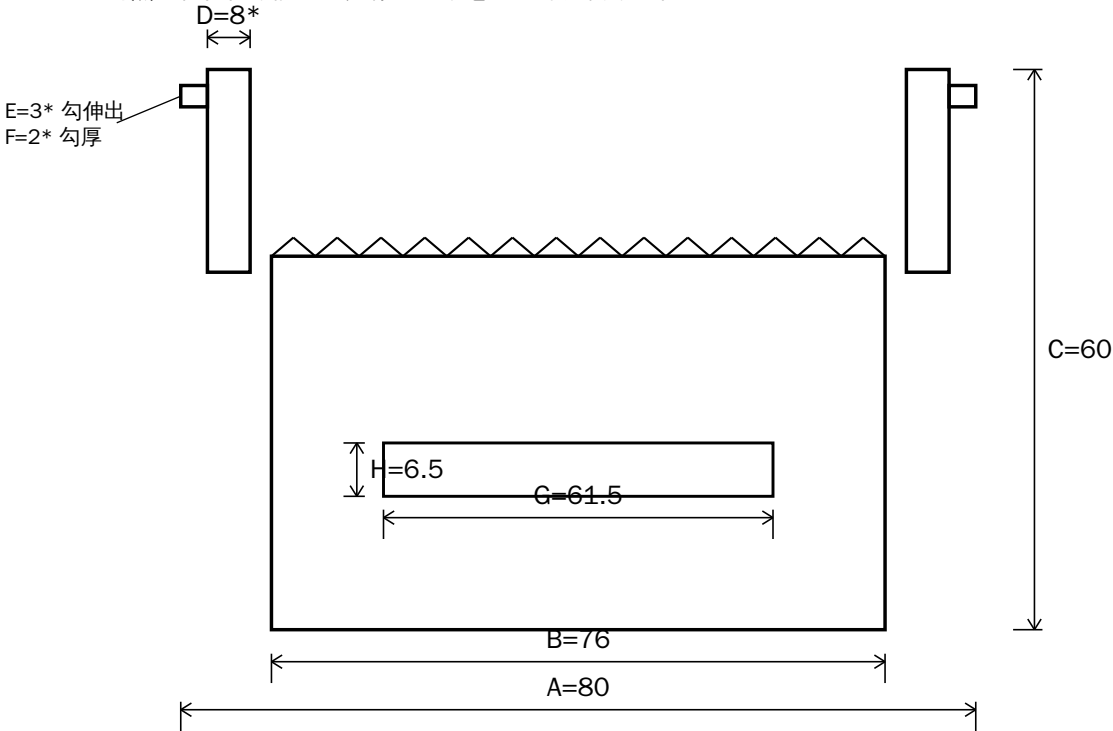
【正面圖】
