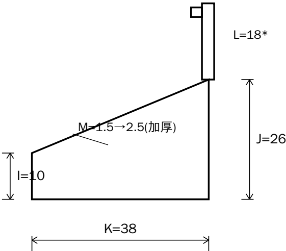
【側面圖】斜角約23°
