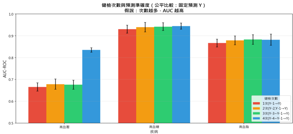
圖 6-7 健檢次數與預測準確度（LR 模型，固定預測 Y）
