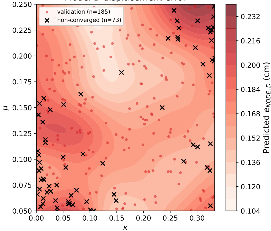
(d) Model D displacement error
