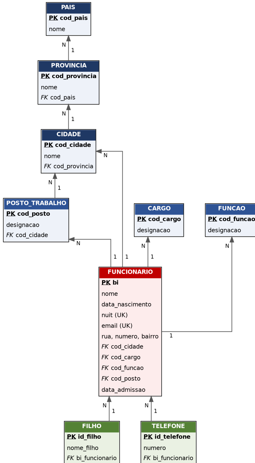
Modelo Entidade-Relacionamento (MER) final — FUNCIONARIO e as suas 8 entidades relacionadas.
