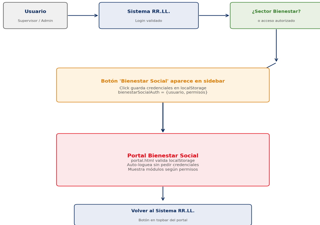
Figura 4: Flujo de integracion SSO
