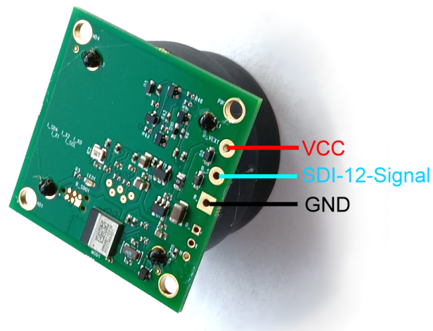
Abbildung 2: PCB-Anschlussvariante mit VCC, SDI-12-Signal und GND
