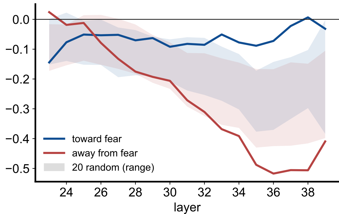
Mistral-24B
