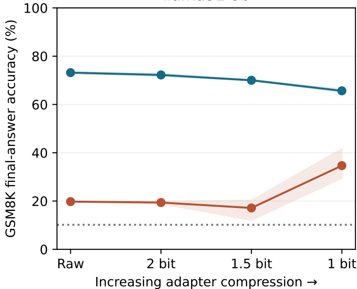
llama31 8b
