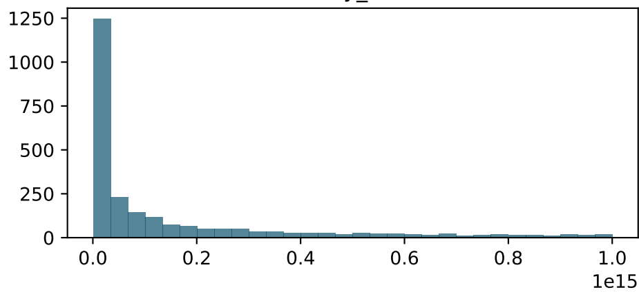
H0
