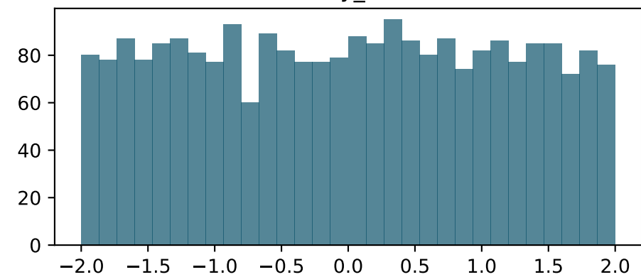
bary_nu
