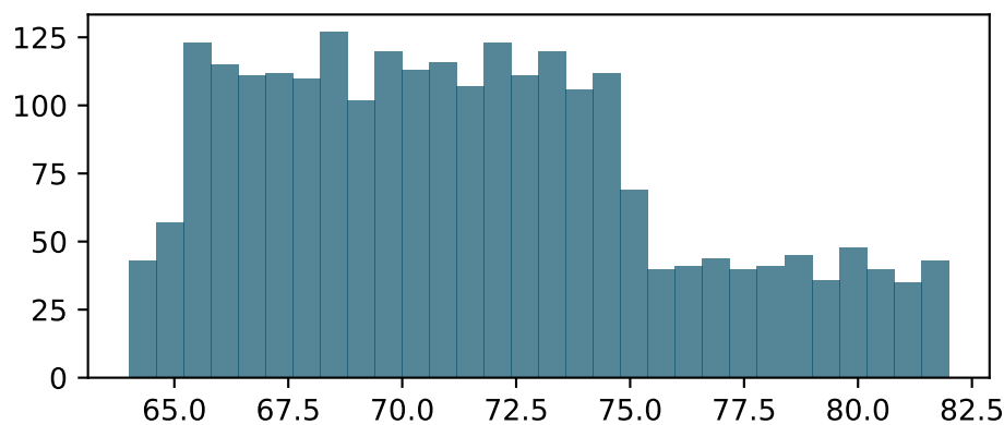
H0
