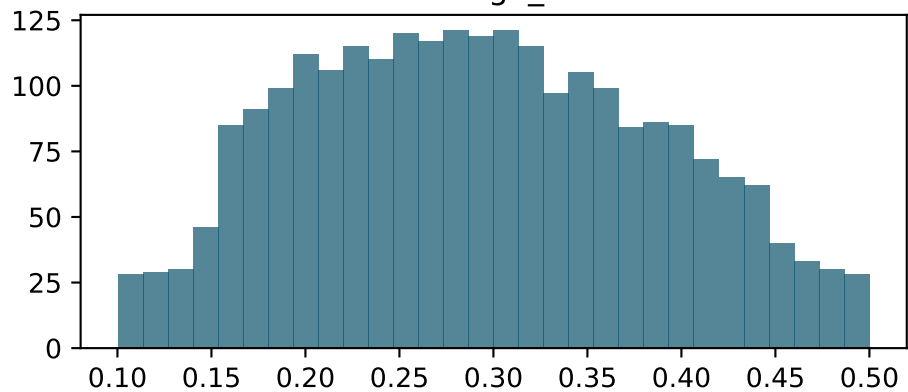
Omega_m
