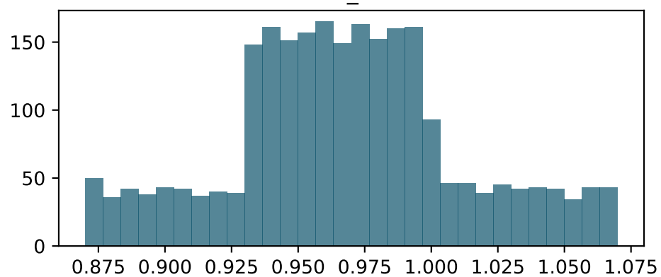
n_s
