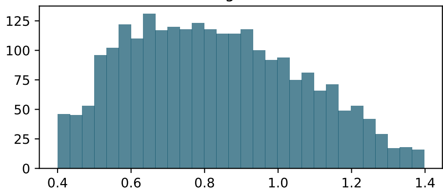
sigma8
