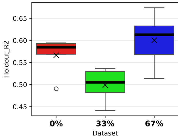
Holdout R^2
