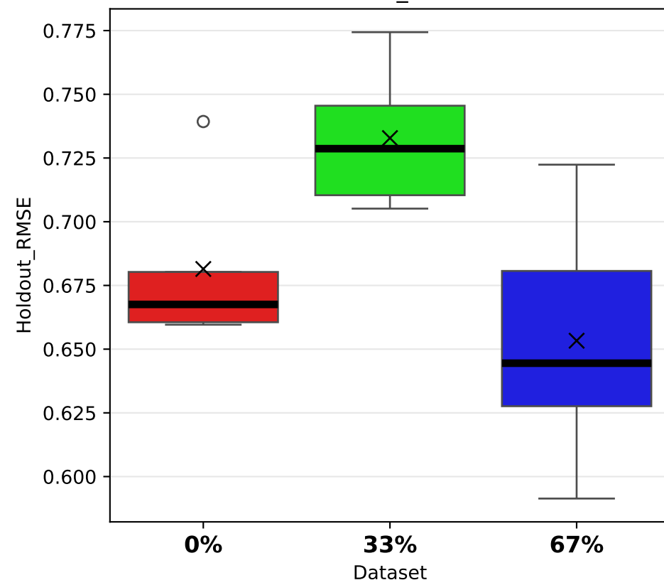
Holdout_RMSE
