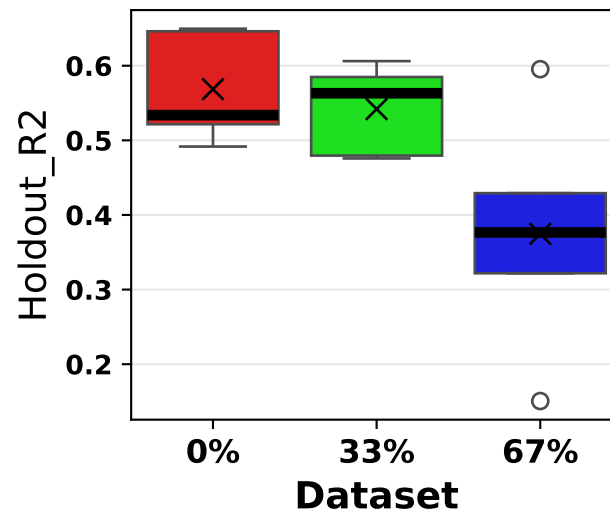
Holdout R^2
