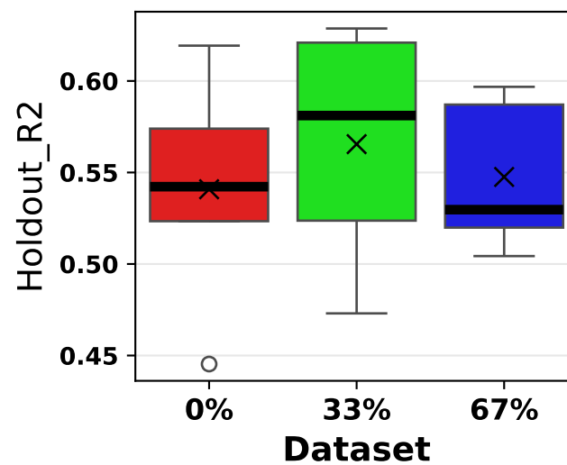
Holdout R^2
