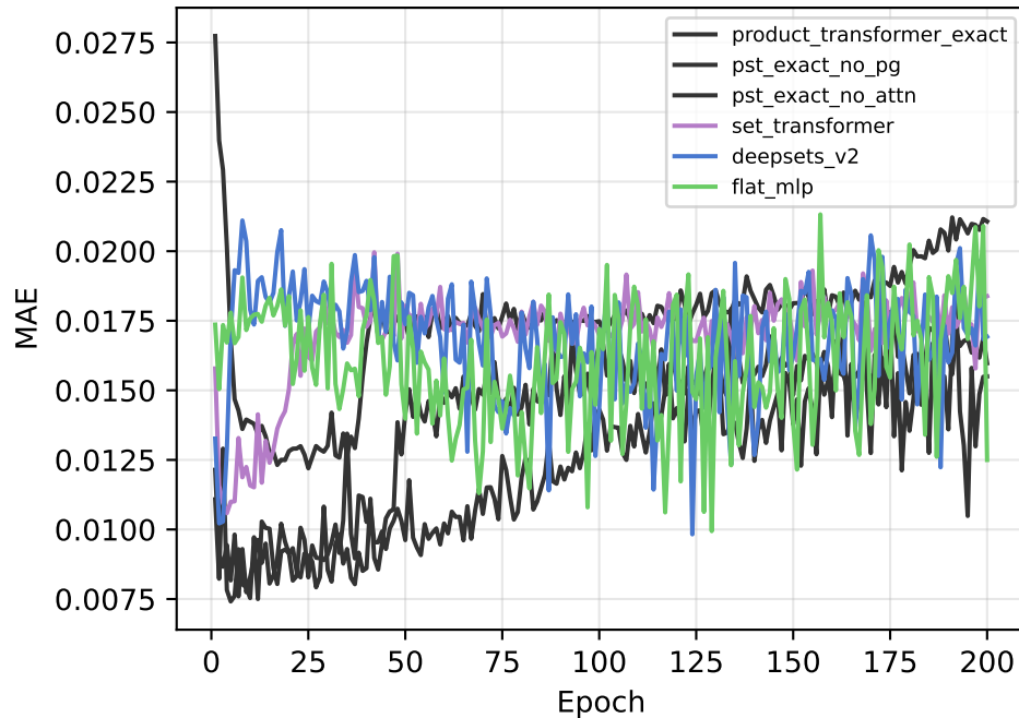
Val MAE
