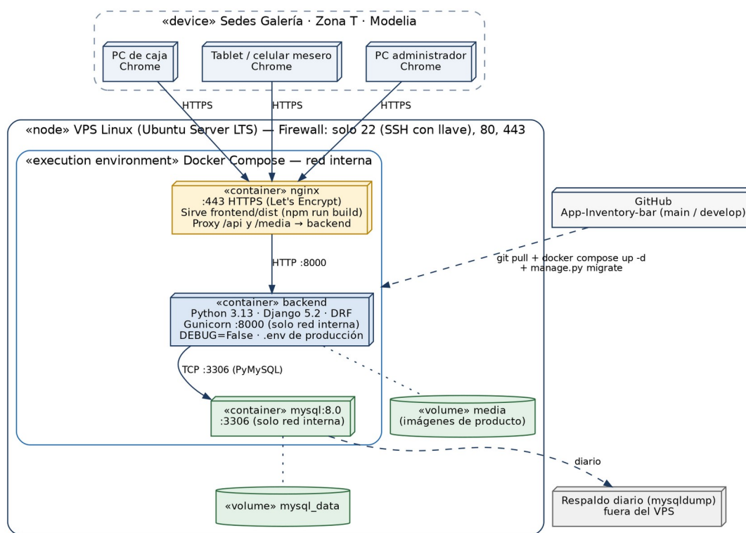
Figura 3. Despliegue en un VPS Linux con Docker Compose.
