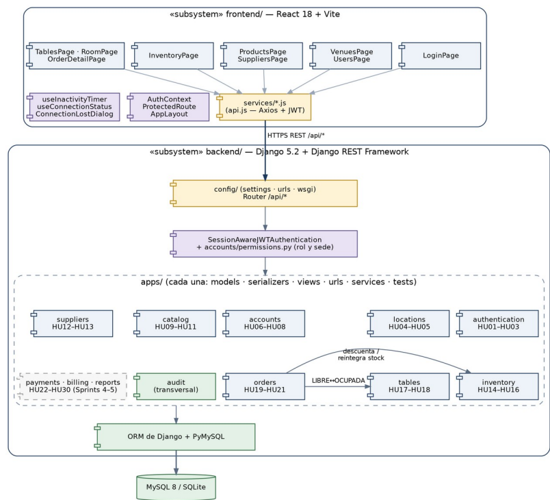
Figura 2. Componentes del frontend y del backend.
