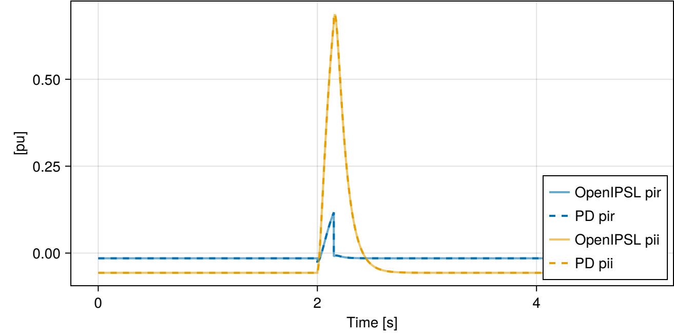
Terminal: pir & pii
