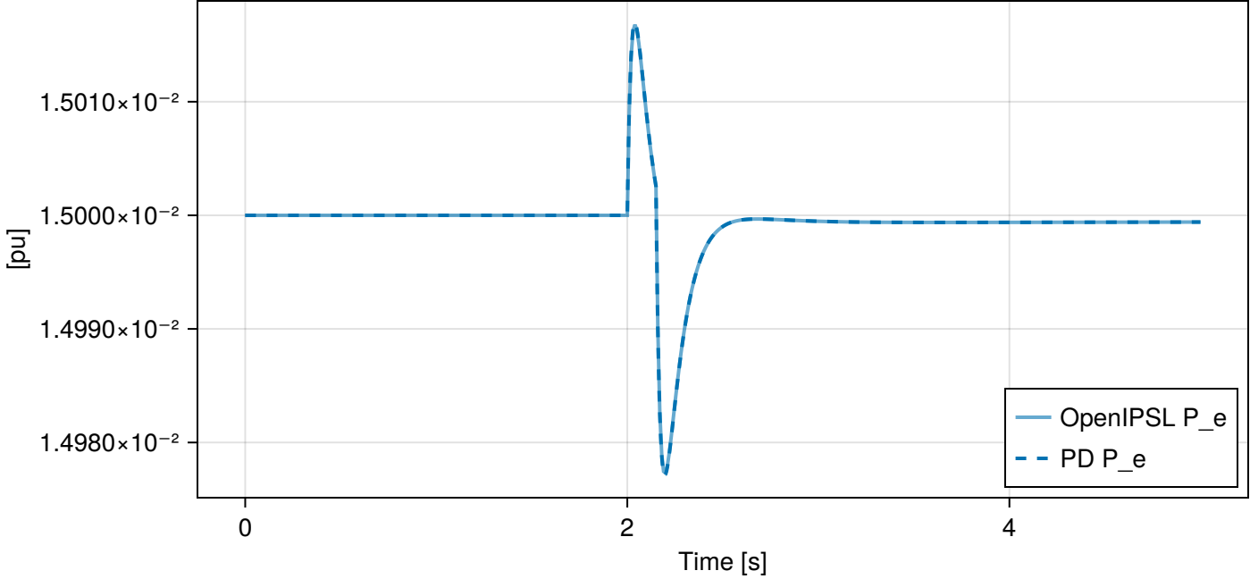
reecb: P_PF (PfFlag)
