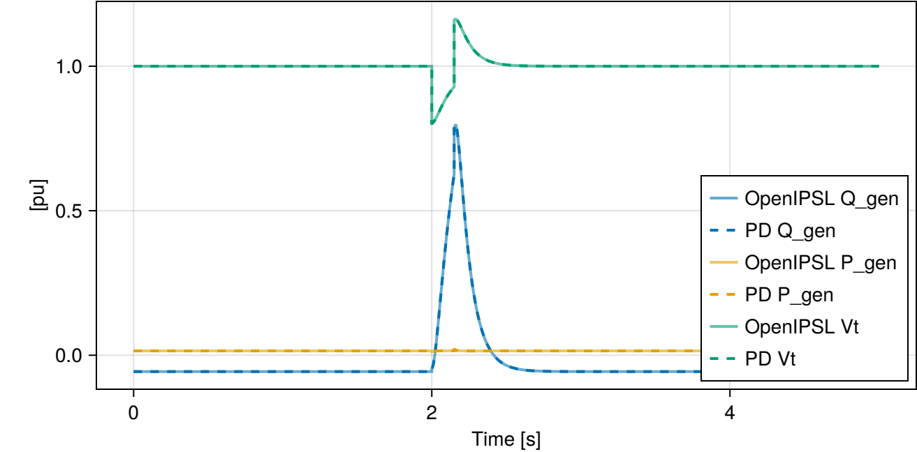
reecb: V_lim & I_lim (QFlag)
