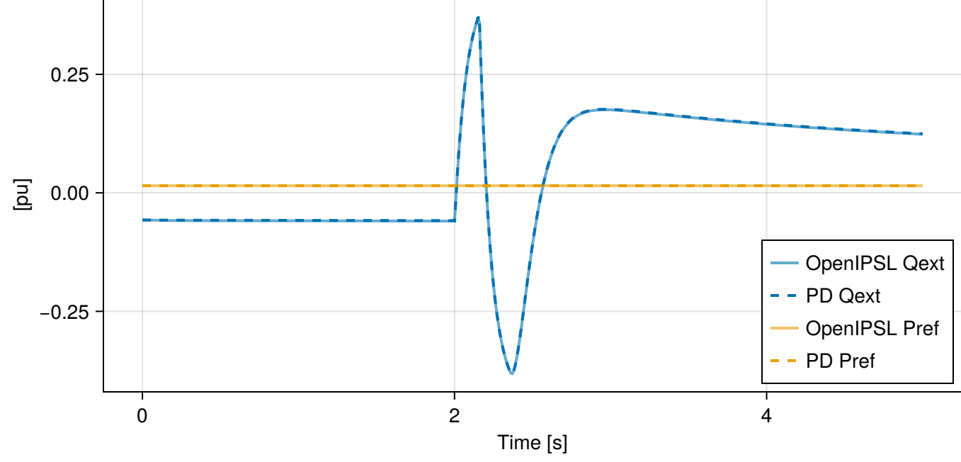
reecb: P_PF (PfFlag)
