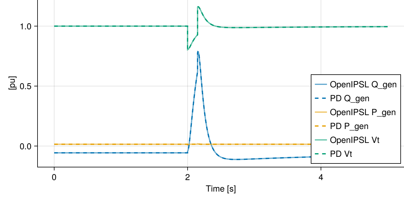
reecb: Q_lim & V_lima (Vflag&&QFlag)
