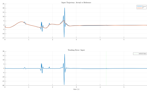
Fig. 9. Inputs: Actual vs Reference
