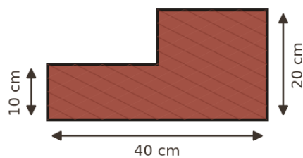
Pieza A.
