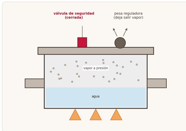
Esquema del funcionamiento normal de la olla · Banco propio IDEA
