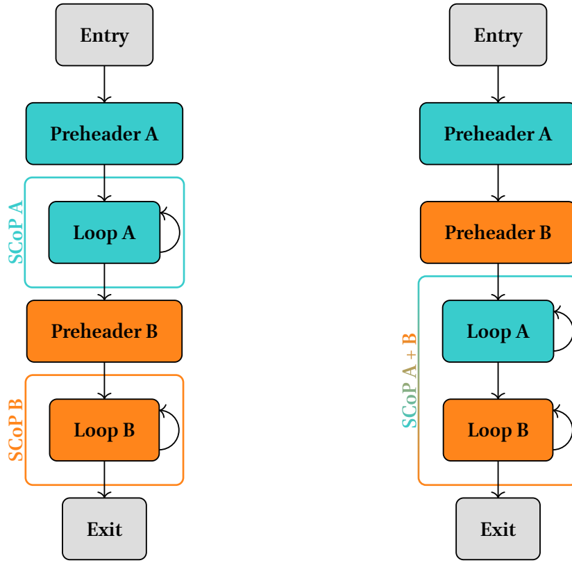
(a) Flot de contrôle initial fragmenté en multiples SCoPs.
