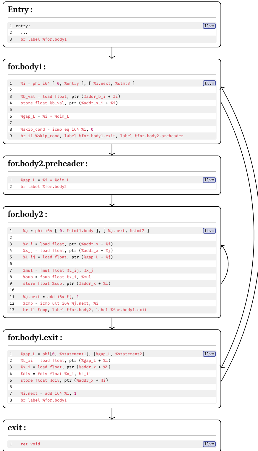
Fig. 15. – Représentation simplifiée en IR LLVM du noyau trisolv (Liste 12).
