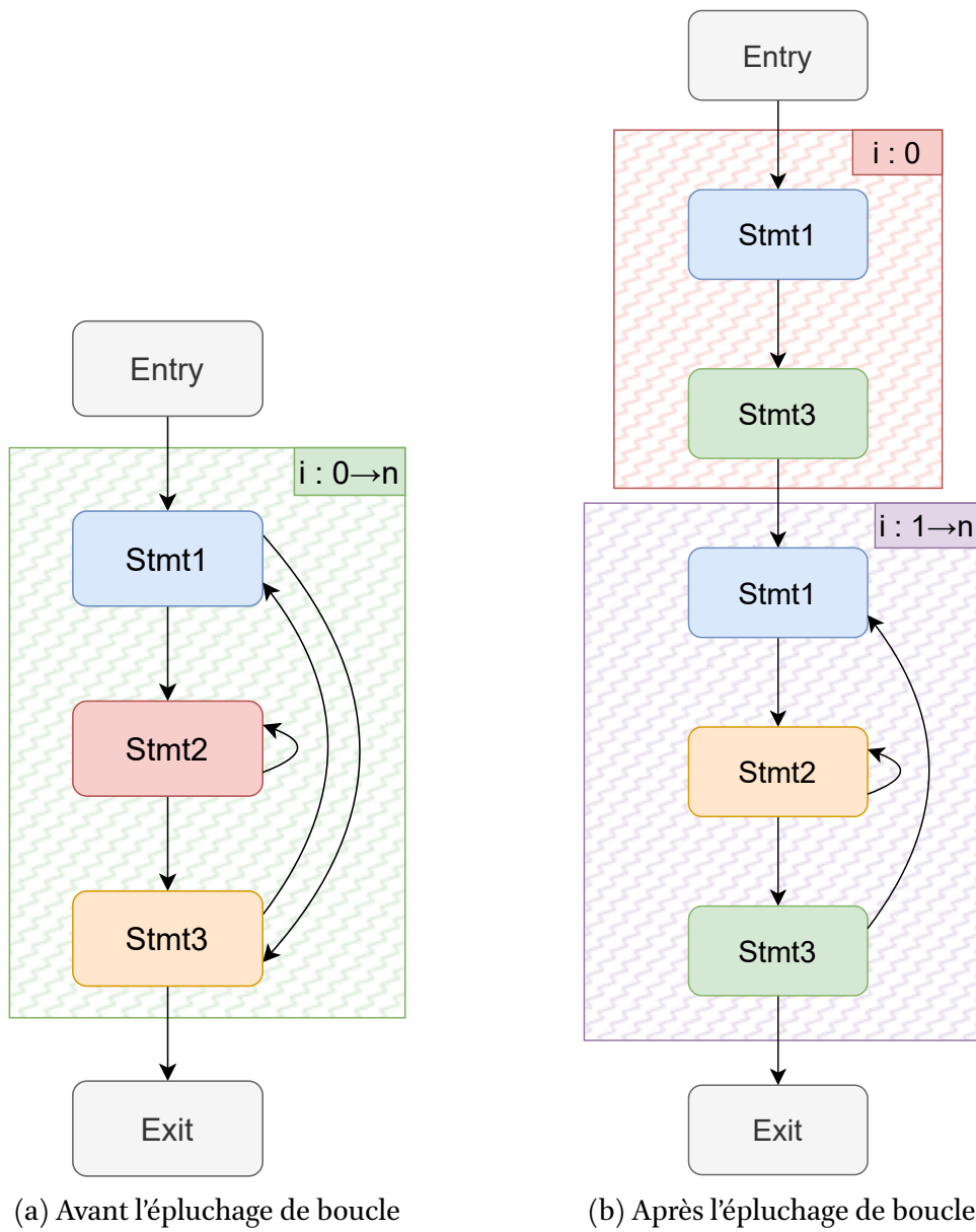
Fig. 16. – Évolution du graphe de flot de contrôle du noyau trisolv suite à la passe d'épluchage statique.
