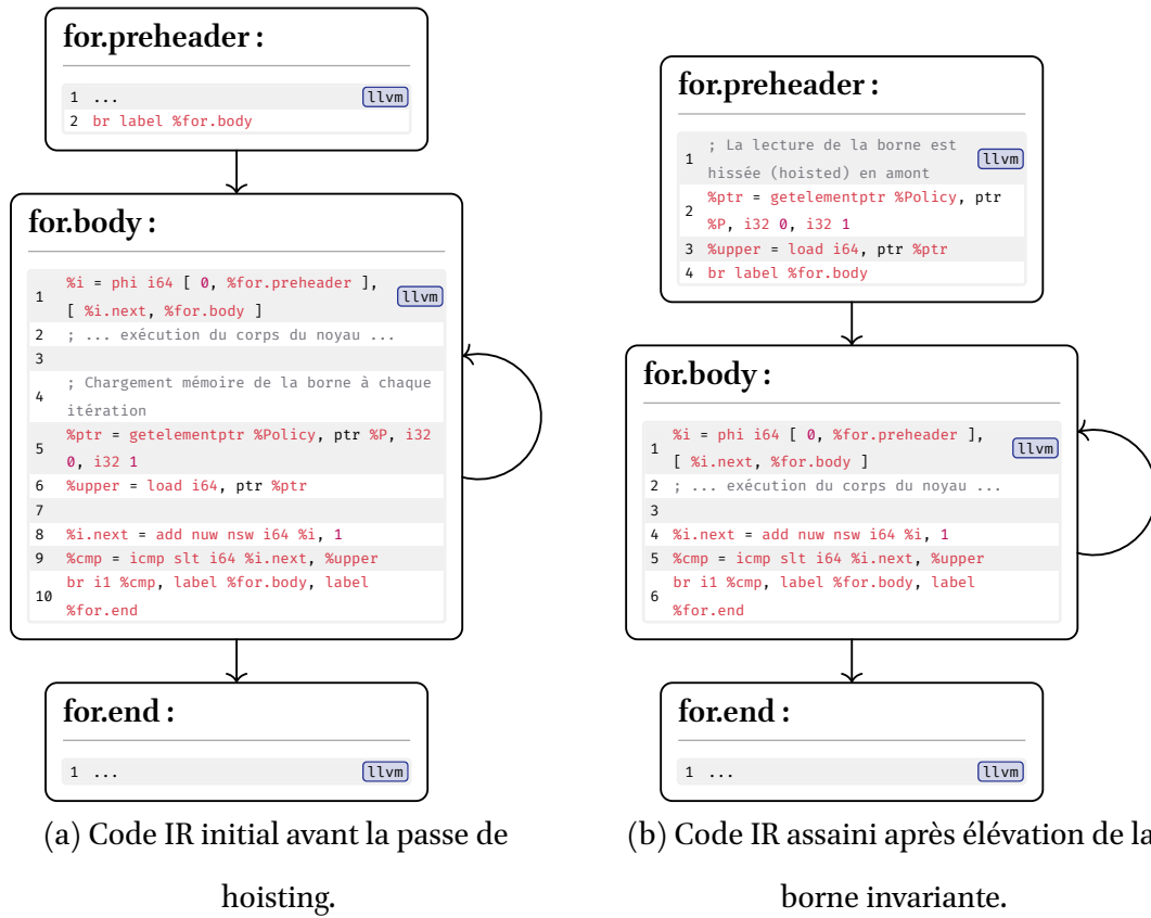
Fig. 10. – Élévation ( hoisting ) du chargement de la borne de boucle dans le pré-en-tête du SCoP.
