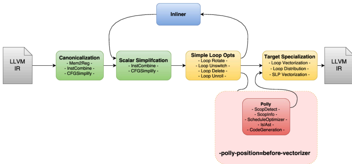
Fig. 4. – Intégration des passes de Polly au sein de la chaîne d'optimisation middle-end de LLVM à la position before-vectorizer . (Source : Documentation de LLVM Polly)
