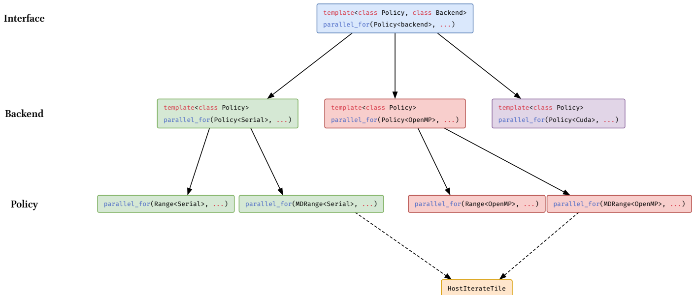
Fig. 9. – Architecture de sélection des backends dans Kokkos.
