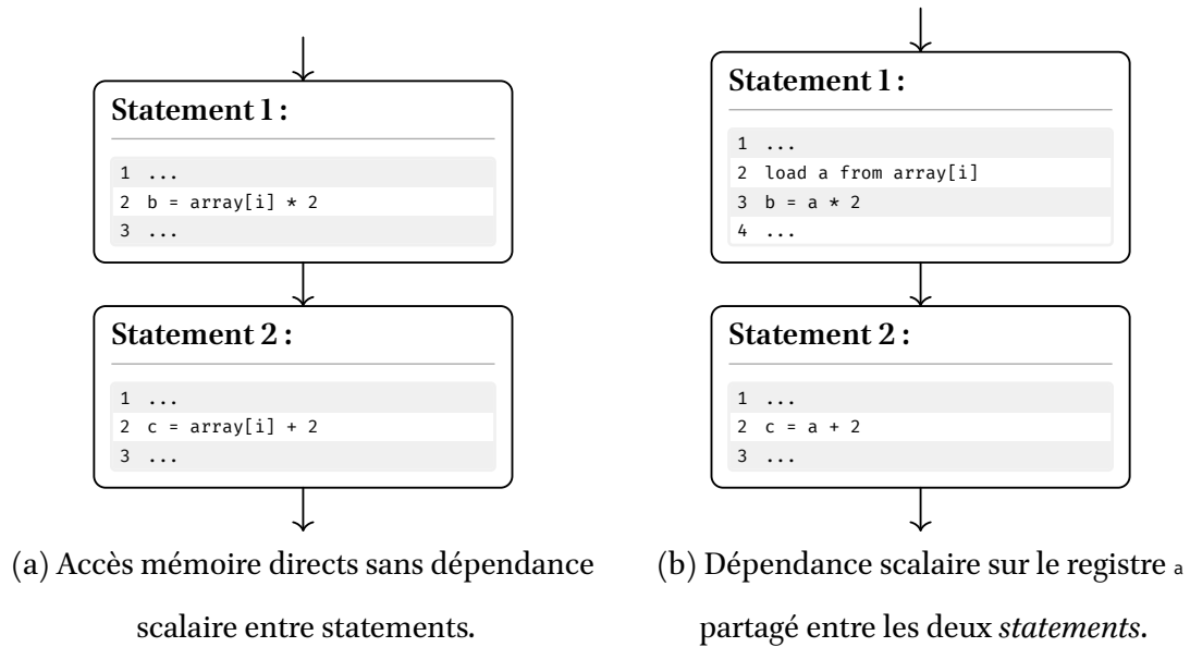
Fig. 12. – Exemple de dépendance scalaire sur a entre deux statements dans le modèle IR de Polly.
