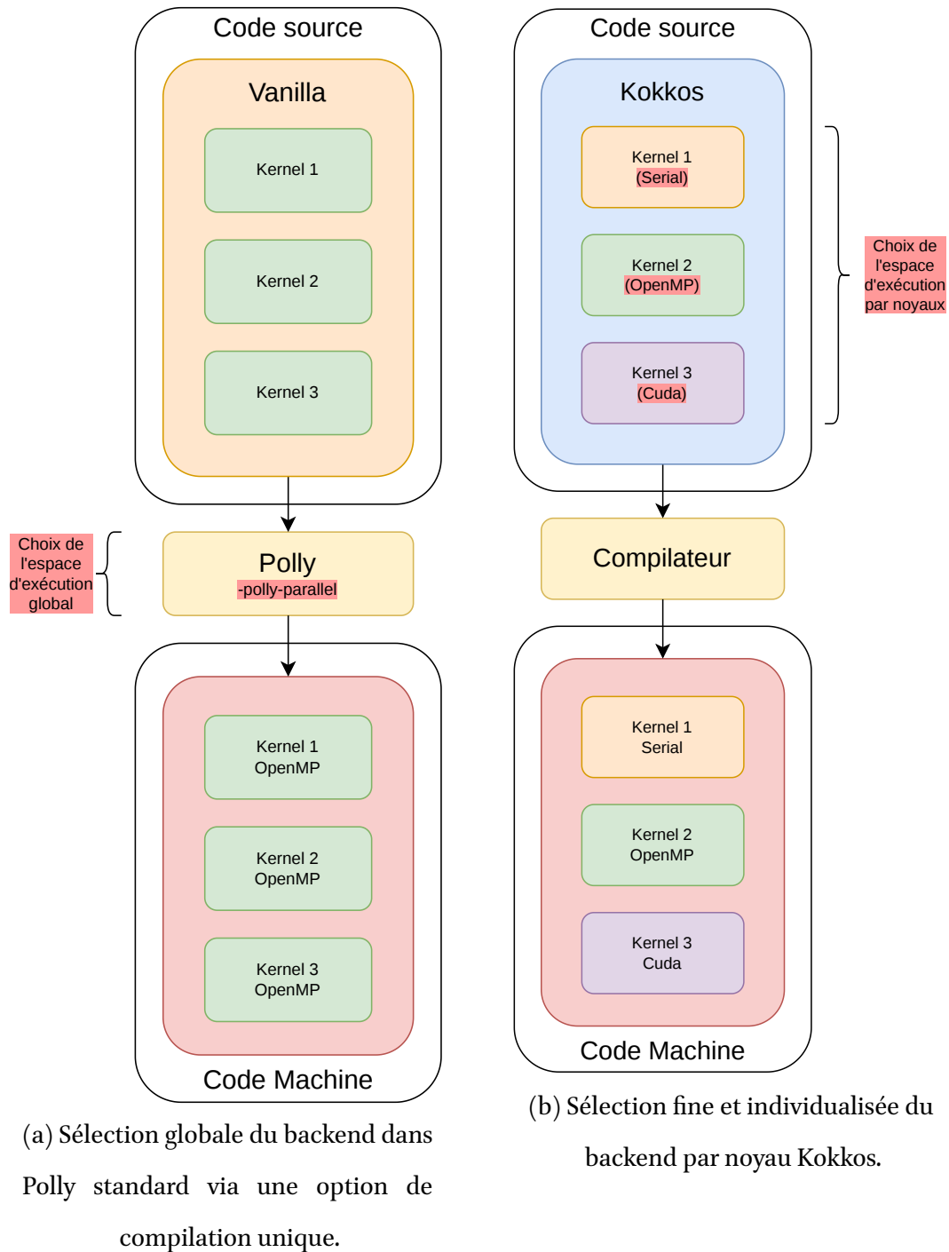
Fig. 14. – Comparaison de la sélection du modèle d'exécution entre l'approche globale monolithique de Polly et l'approche fine par noyau de Kokkos.
