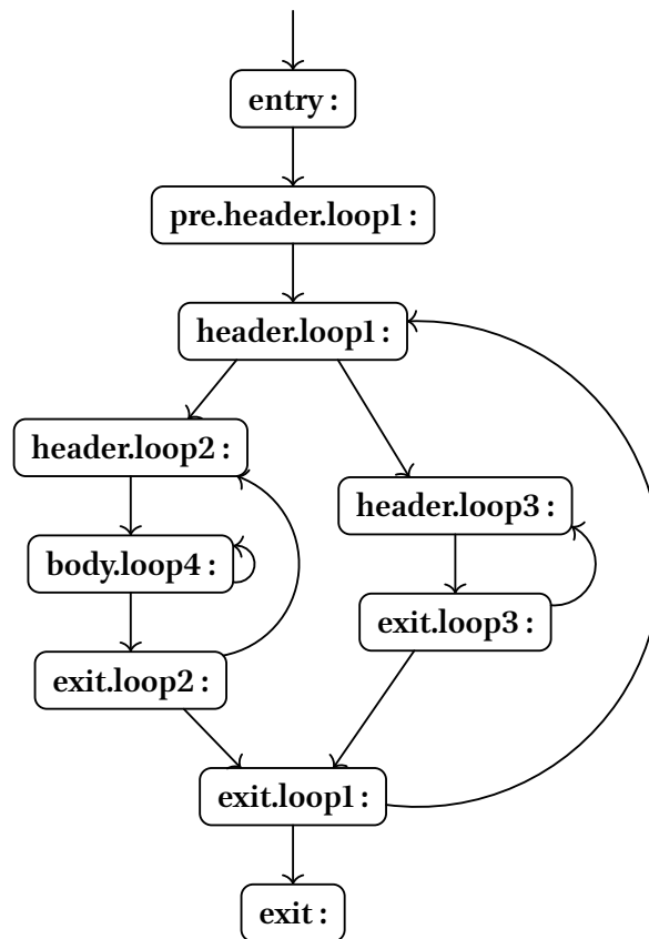
Fig. 11. – Exemple de graphe de flot de contrôle (CFG) complexifié par des branchements conditionnels et du versionnage de boucles, entravant la détection du SCoP.
