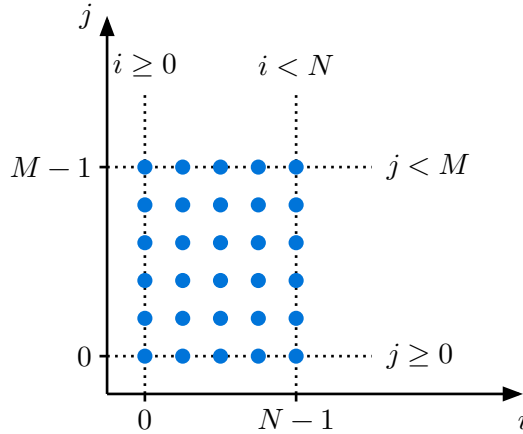
Fig. 1. – Représentation géométrique du domaine d'itération pour l'instruction S_1 .
