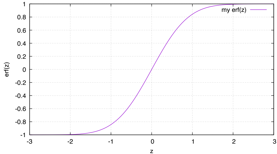
Error Function
