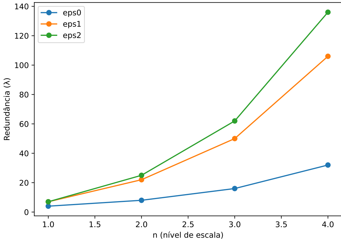
Resultados (Results-Only): Redundância ( \lambda ) vs n
