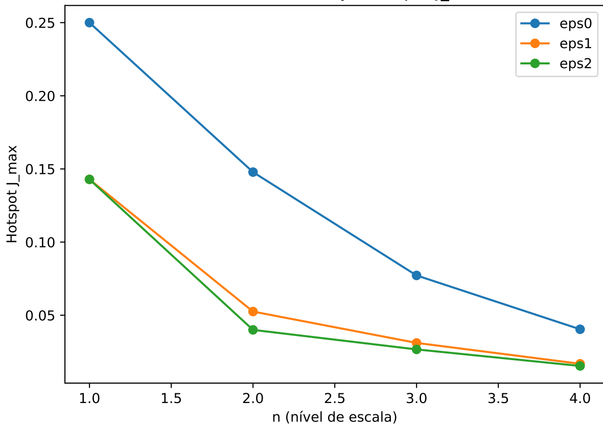
Resultados (Results-Only): Hotspot J_max vs n
