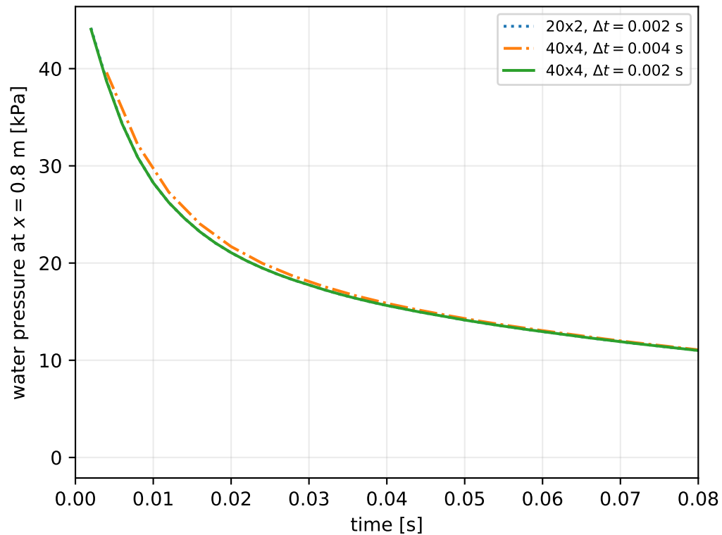
Drainage-front refinement
