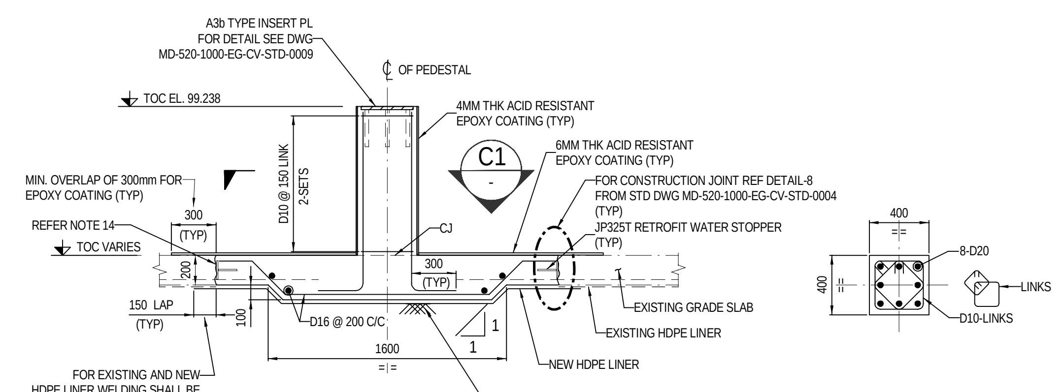
SECTION C-C (SCALE: 1:25 mm)
