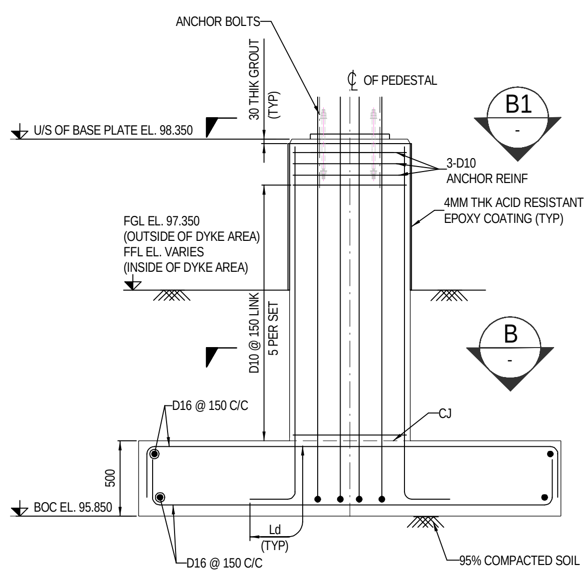
SECTION A-A LOOKING WEST (SCALE: 1:25 mm)
