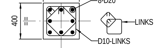
SECTION C1-C1 (SCALE: 1:25 mm)
