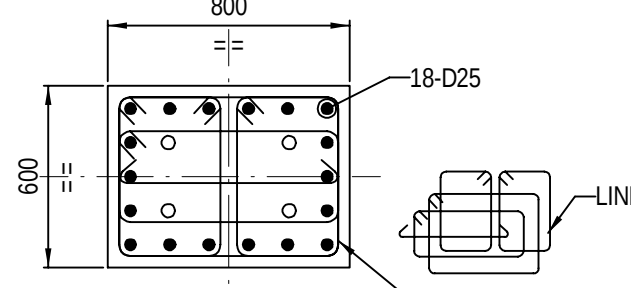
SECTION B-B (SCALE: 1:25 mm)
