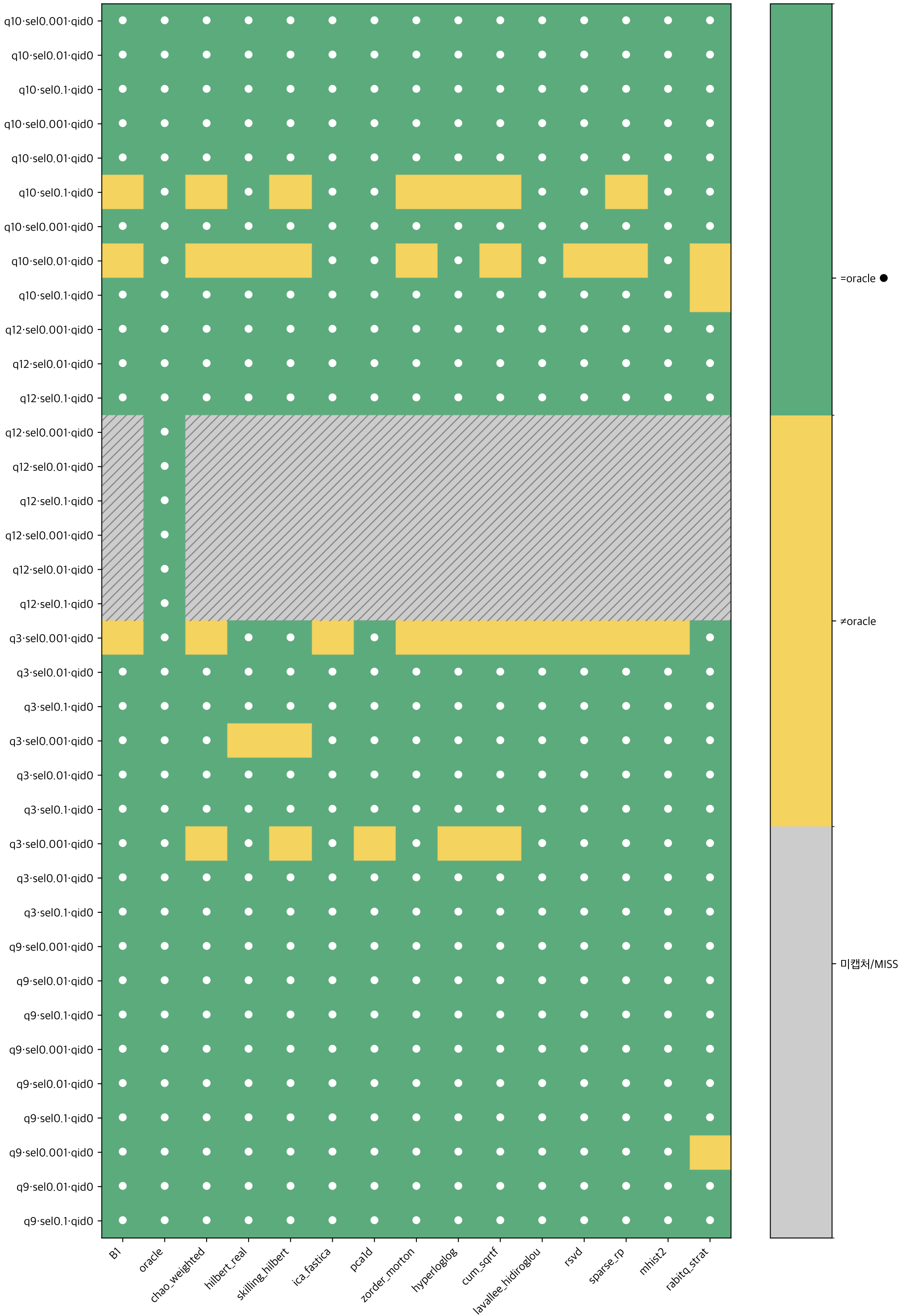
실행 계획 회복 — oracle 과 동일 plan 여부
